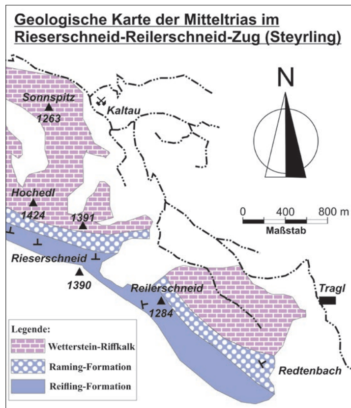
ABB. 20: Geologische Karte Kaltau FIG. 20: Geological Map Kaltau
